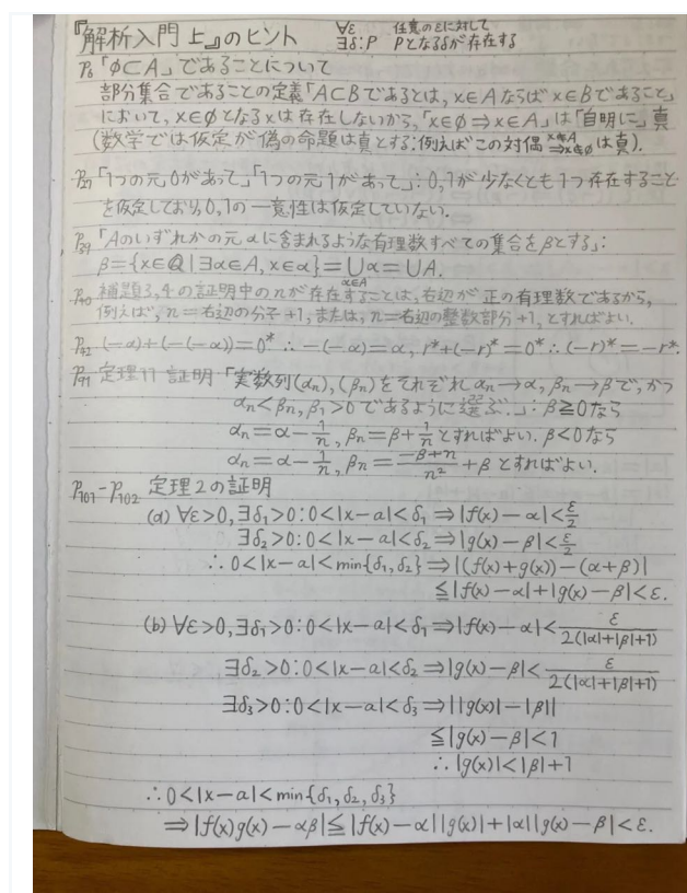
極限の性質. 和(積)の極限は極限の和(積)
